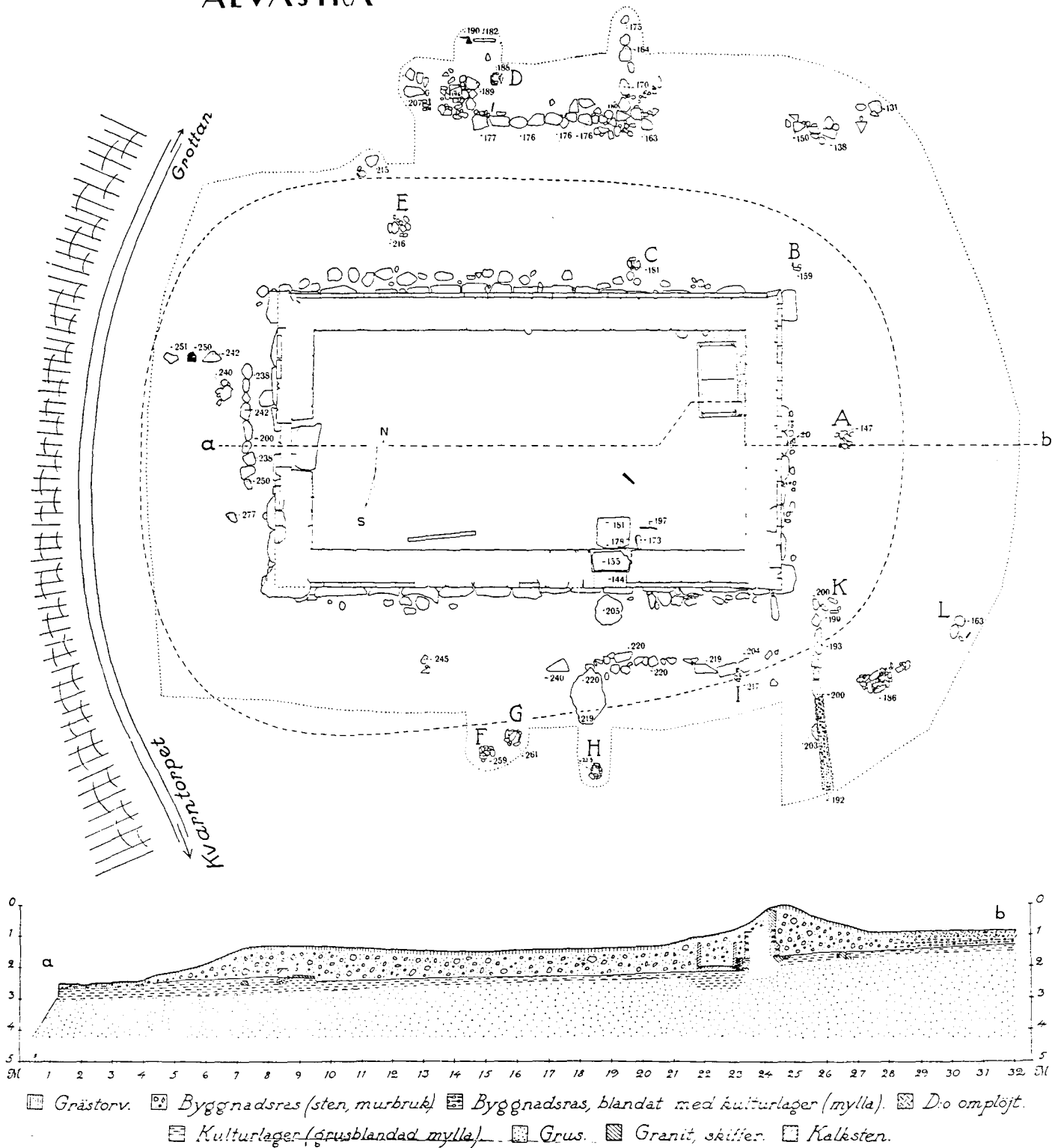
Fig. 50. "Sverkerskapellet", Alvastra; plan och skärning. Vid A—L stolphål; ----- ruinkullens omkrets; ..... gräns för det undersökta området.
